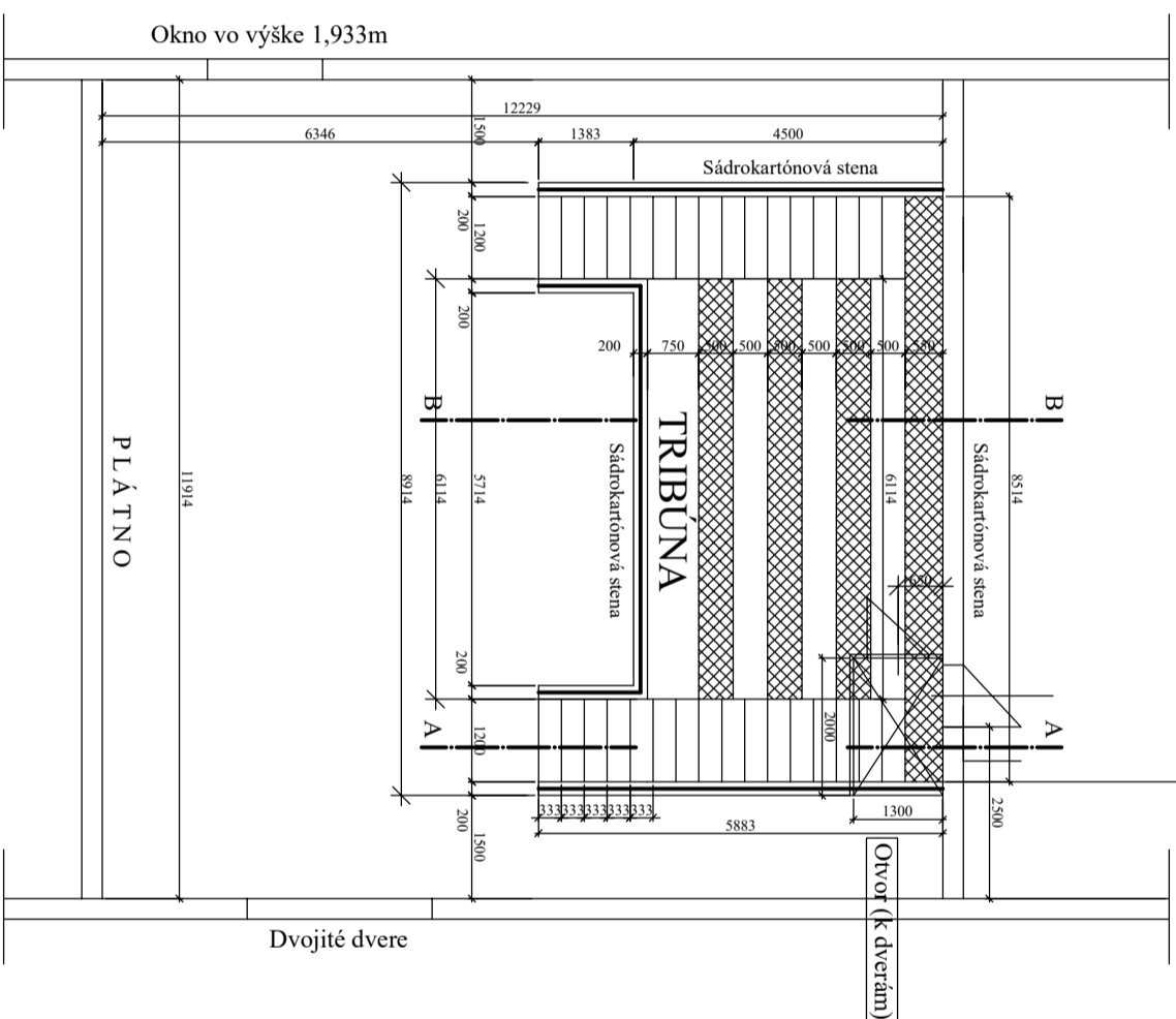
PODORYS
